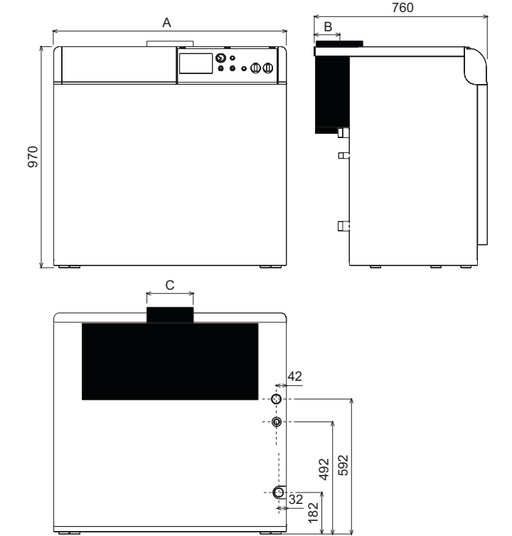
рис. 13 - Габаритные размеры и присоединения
