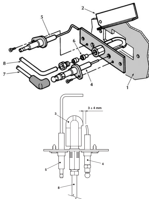
рис. 11 - Пилотная горелка
